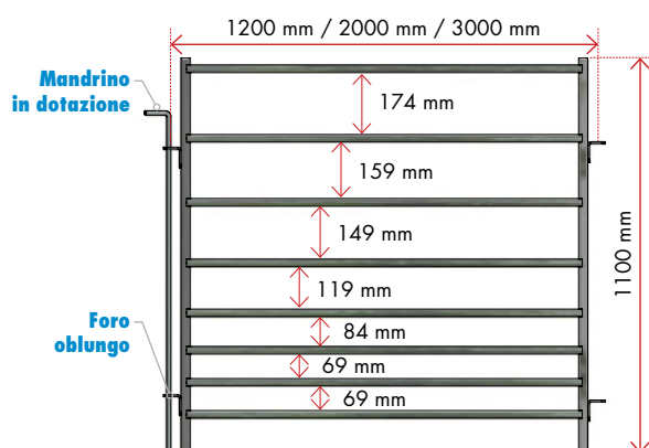
Versione singola a 8 tubi :
