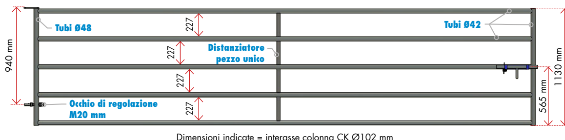
Occhio di regolazione M20 mm con foro Ø16 mm
