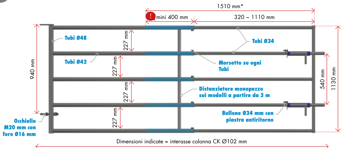
Versione con porta a catenaccio singolo
