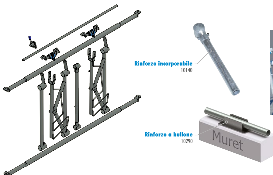
Antiribaltamento della testa Serranda da montare sul lato animale.
