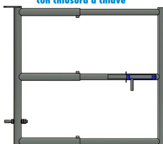
Versione standard della porta con chiusura a chiave
