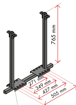
Supporto per corridoio
