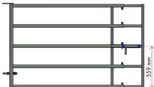
Versione con porta a catenaccio singolo
