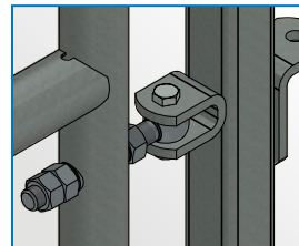
Occhiello Ø20 mm per la regolazione del livello
