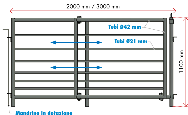
Versione singola a 8 tubi :
