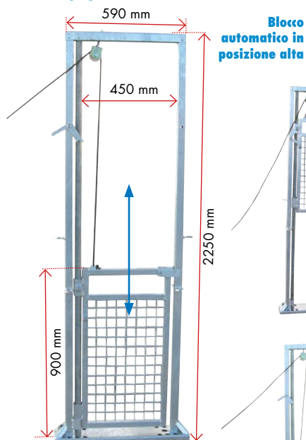
Porta a ghigliottina
