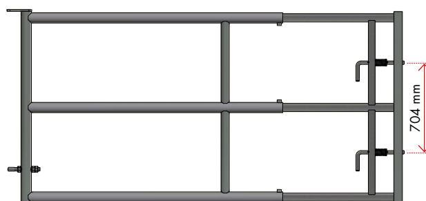
Versione con porta a molla
