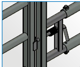
Puerta peatonal incorporada con pestillo de resorte para cierre automático
