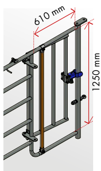
Puerta peatonal reversible con gancho para mantenerla en posición abierta
