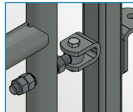
Ojal de Ø20 mm para ajuste de nivel
