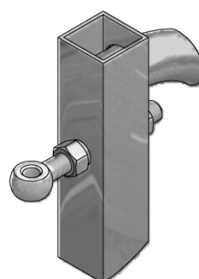
Ojales ajustables 52199 et 10199
